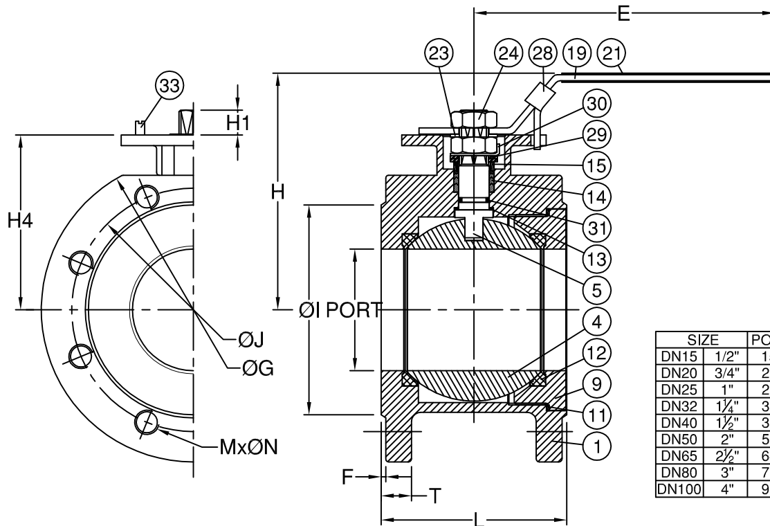
DN15~DN25 BODY
