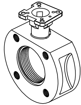
DN15~DN25 BODY
